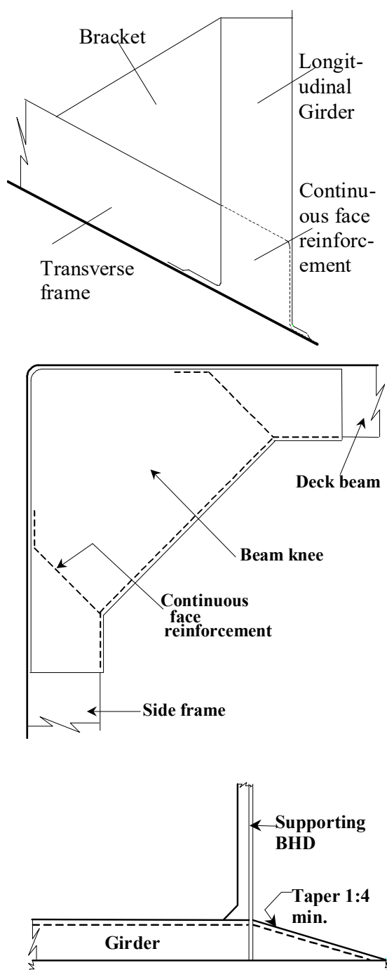
Fig. 1.5.1 : End attachments
