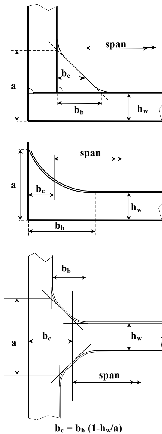
Fig. 1.4.2 : Girder end details
