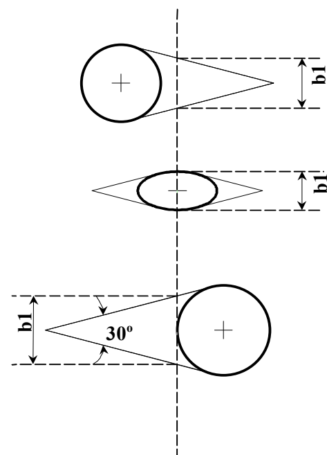
Fig. 2.3.1 : Shadow areas
