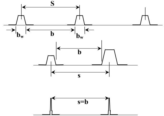
Fig. 7.3.2 : Panel dimensions
