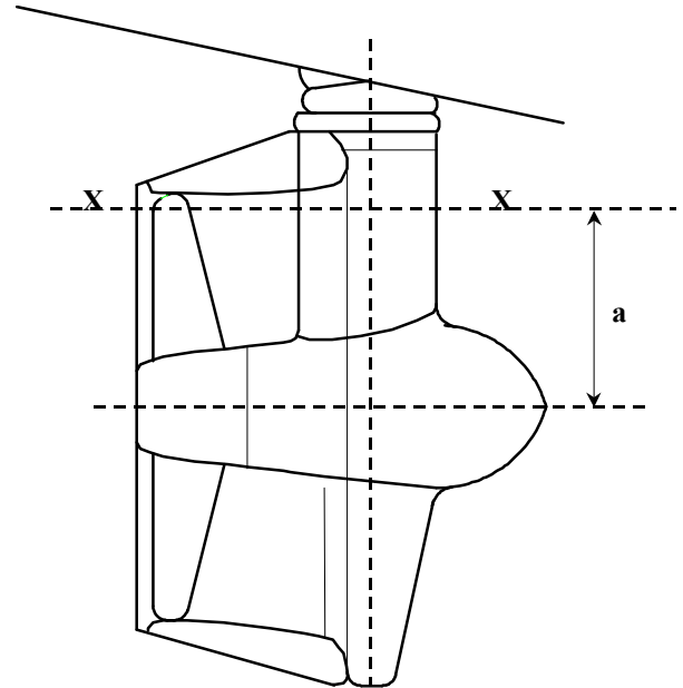
Fig. 4.2.4.3.2 : Azimuth thruster
